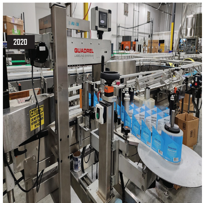
2020 Quadrel Techline Q120 WRAP Labeling Machine.
