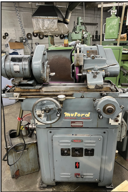
MYFORD PRECISION OD GRINDER, S/N S 85894 -CB.
